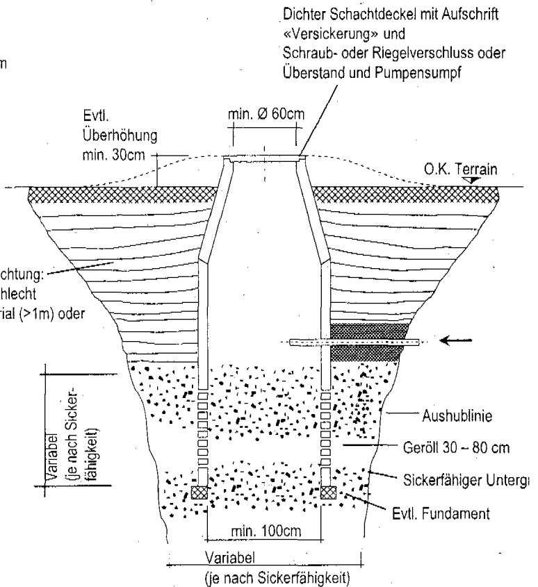
Beispiel Sickerschacht
