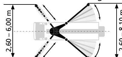
iSC – Flexible Abstützung
