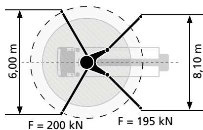
Standard – Vollabstützung
